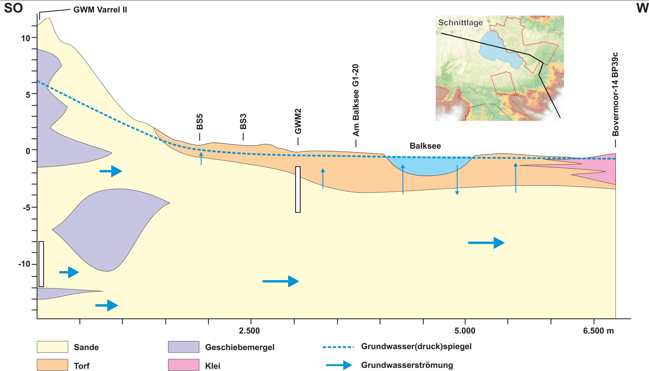
Anl. 5: Hydrogeologischer Schemaschnitt
